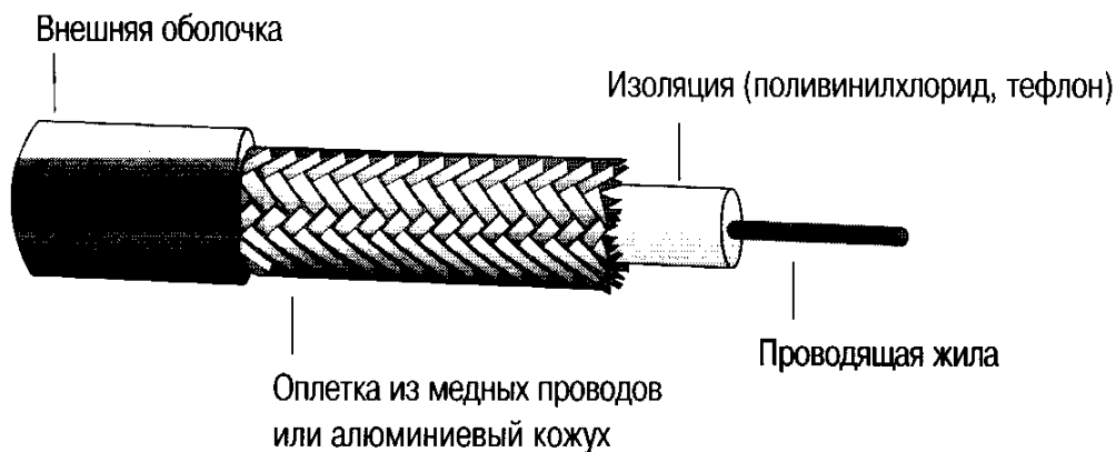
Сурет 1. Коаксиалды кабельдің құрылымы
