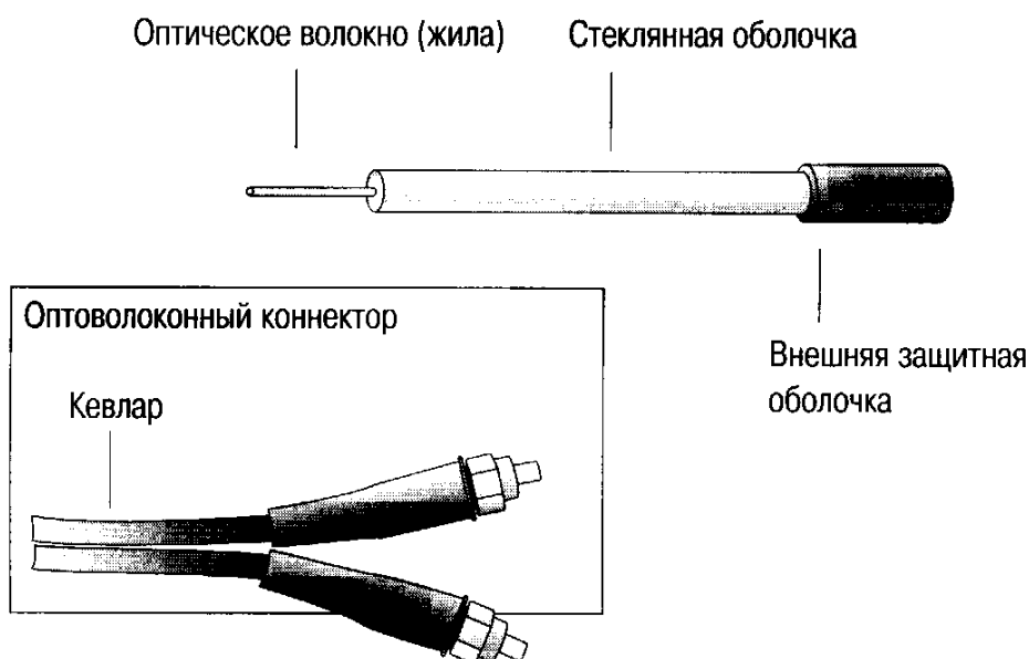
Сурет 14. Оптикалық талшықты кабель
